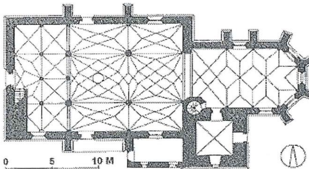
Grundriss der Pfarrkirche Haidershofen
